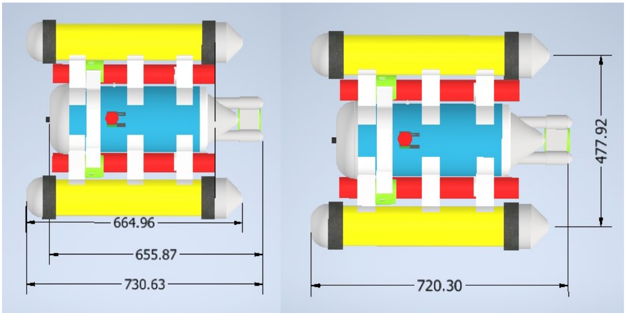
Gambar 28. Tampak Atas
