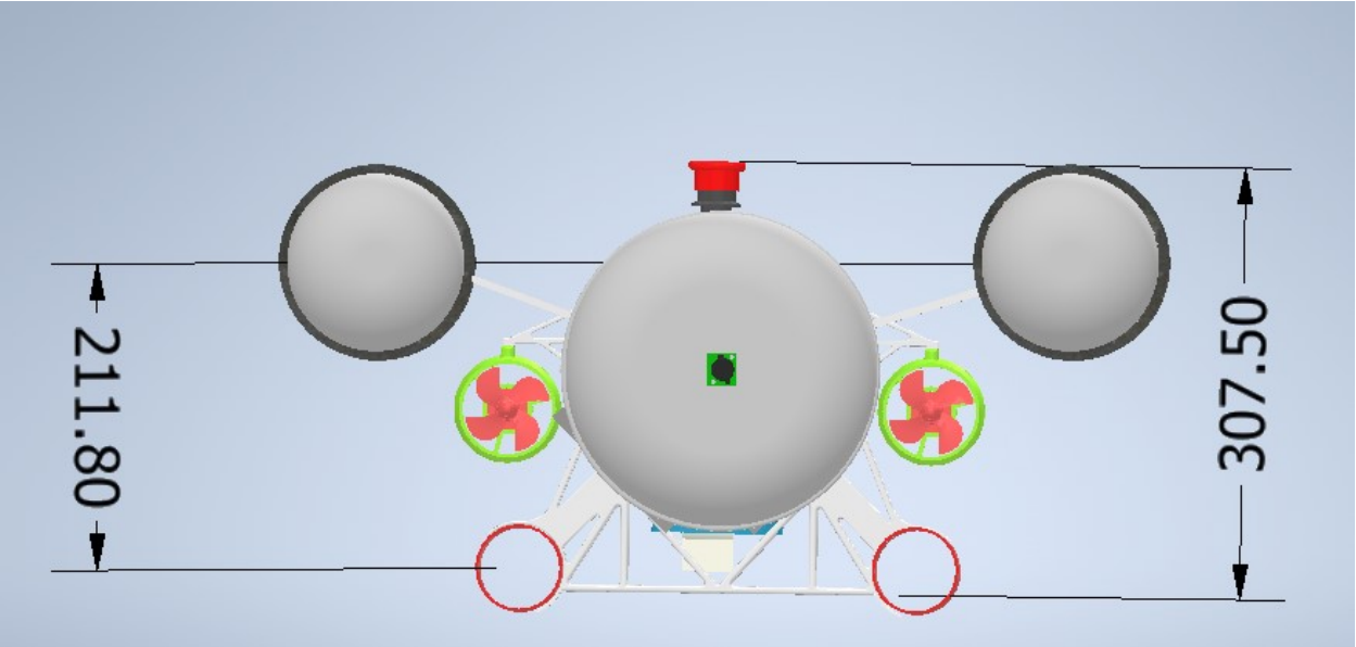
Gambar 29. Tampak Depan
