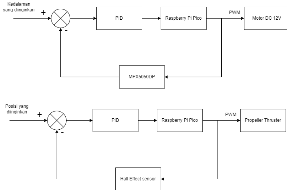
Gambar 3.1: PID robot
