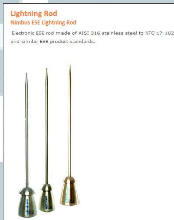
Gambar 2. 8 Lightning Rod Nimbus ESE Lightning Rod
