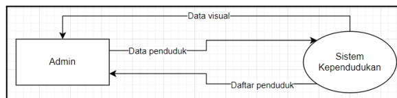
Gambar 3.2 DFD Level 0
