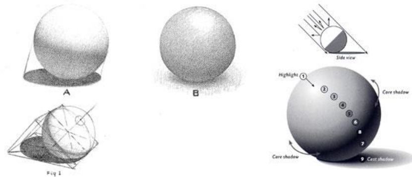
Gambar 2.6. Specular
