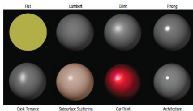
Gambar 2.9. Tipe-Tipe Shader
