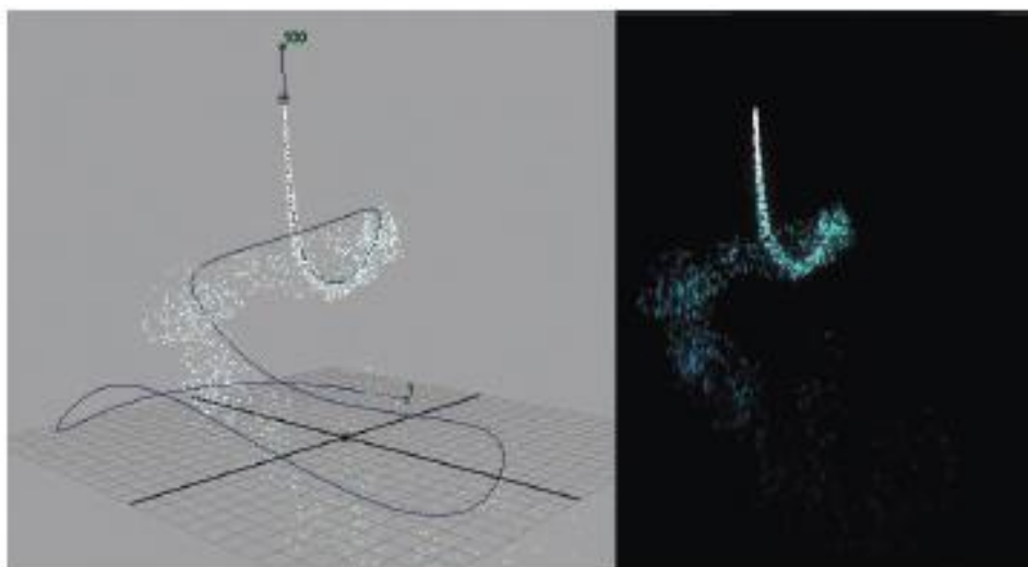
Gambar 2.12. Particles
